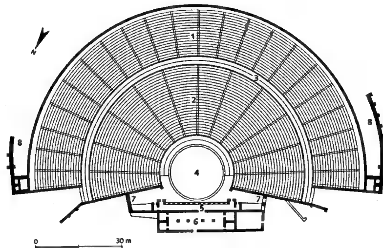
Epidauros, Theater; 2. H. 4. Jh. v. Chr. (Grundriß). 1 jüngeres kōilon 2 älteres kōilon 3 diázōma/Gürtelgang 4 orchēstra/Spielfläche 5 proskēnion/Bühne 6 skēnē/Bühnengebäude 7 pártodos/seitlicher Zugang 8 Stützmauer
